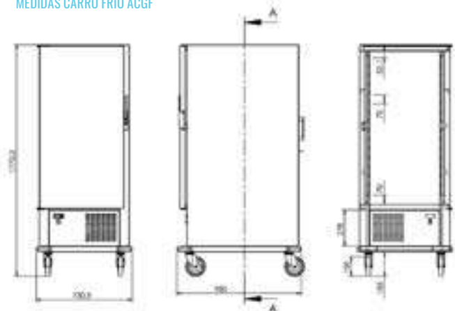
MEDIDAS CARRO FRÍO ACGF
