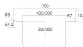
MEDIDAS CUBETA
