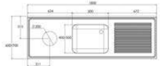
MEDIDAS FREGADERO 1800 MM
