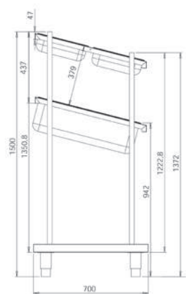
MEDIDAS DISPENSADOR
