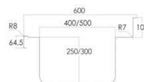
MEDIDAS CUBETA
