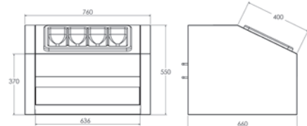
MEDIDAS DISPENSADOR
