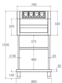
MEDIDAS DISPENSADOR
